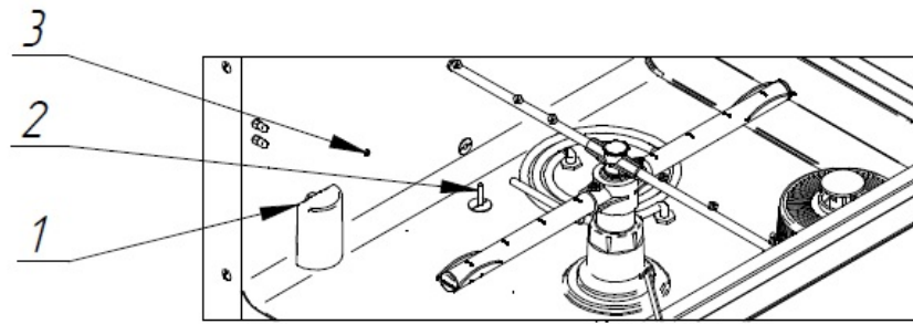
1 Воздушная камера; 2 Датчик температуры ванны; 3 Отверстие для подачи моющего средства
